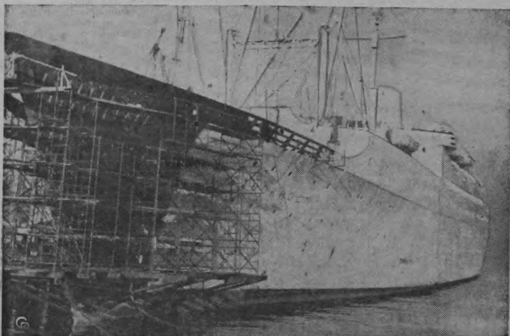
El barco de pasajeros sueco Stockholm aparece al ser sacado del astillero en Brooklyn, Nueva York, y trasladado a un nuevo muelle. Andamios especiales aun cubren la nueva proa que se le ha hecho y que ha costado $ 900.000.00 reparación necesaria como resultado del desastroso choque en el Atlántico con el Andrea Doria el pasado julio.—(INP). F
